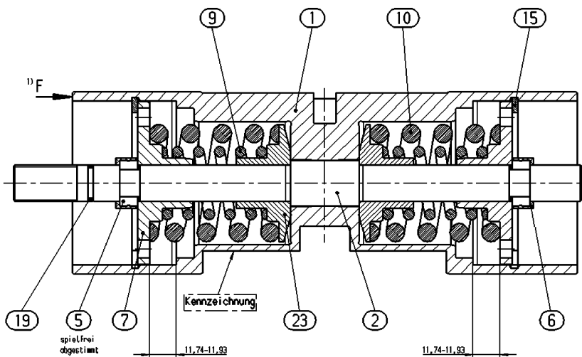
1) Stellkolben, komplett
