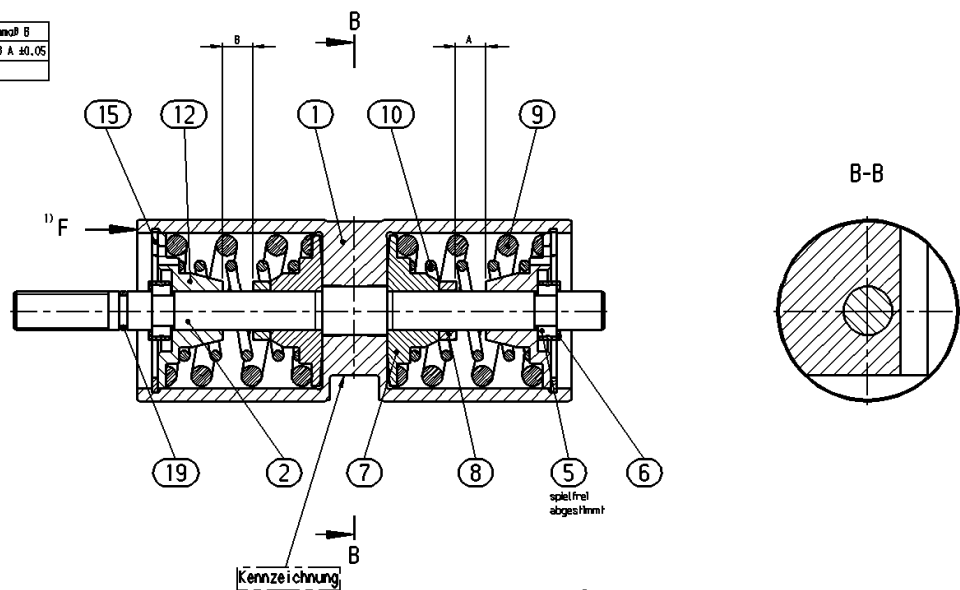
1) Stellkolben, komplett
