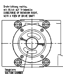
A-A 1:2,5
