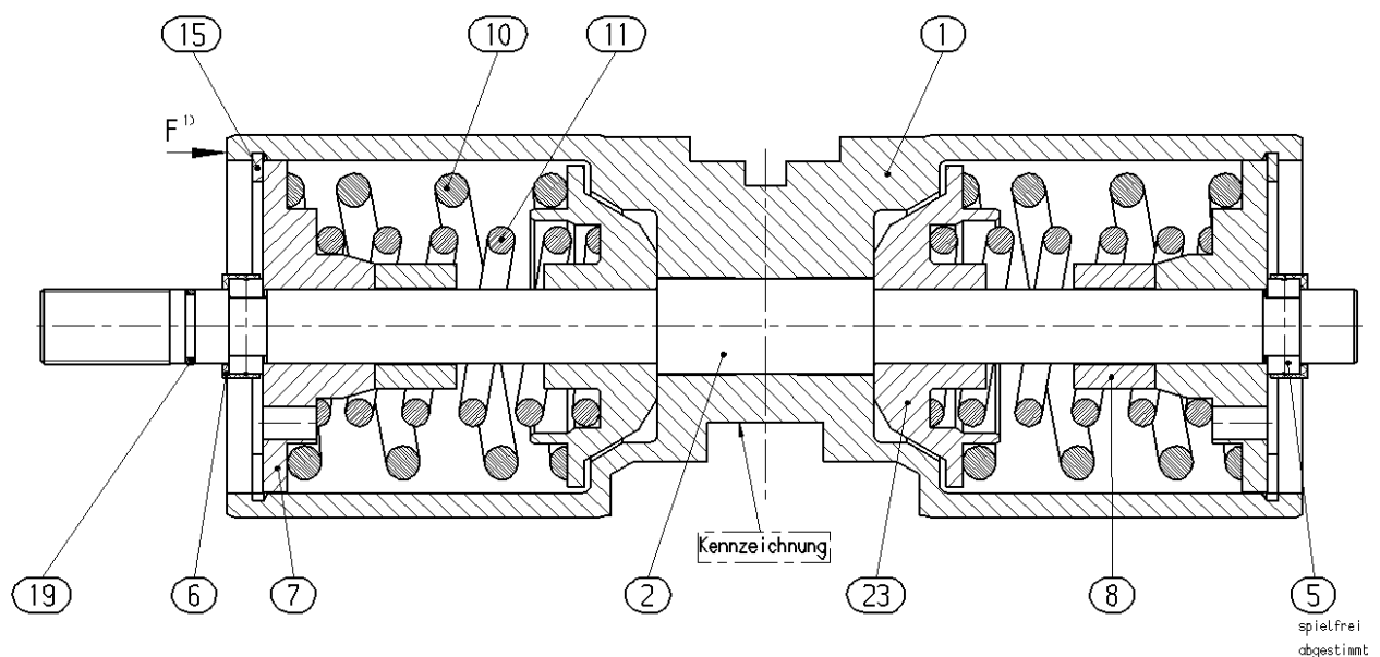
1) Stellkolben, komplett
